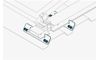
Trapezblechadapter zur einfachen Anbindung an Trapezblechdächer
