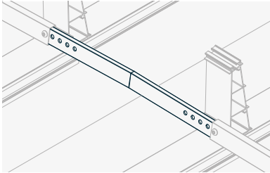
Firstkopplung in Modulrichtung
