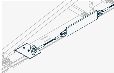
Absturzsicherung zur Sicherung von einer Person gegen Absturz
