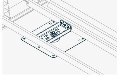
Solmont-Montagefuß und USO-Anbindung zur sicheren Anbindung der Anlage auf dem Dach und/oder zur Ballastreduktion
