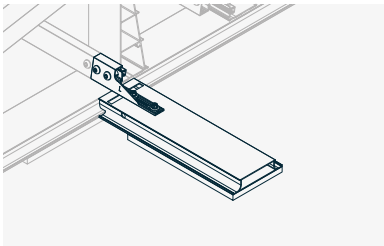
Trassierung mittels systemabgestimmter Bauteile inkl. der Integration im Blitzschutzkonzept und des Potentialausgleichs
