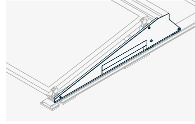
Seitendeckel zur Verbesserung der Aerodynamik und Reduktion des Ballastes
