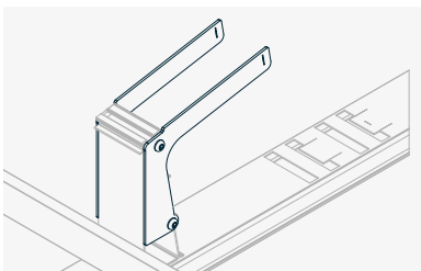
Mittelabstützung zur Modul- und Dämmungsentlastung
