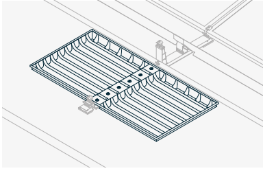
Ballastwanne als Alternative zu Ballaststeinen für bekieste und begrünte Dächer
