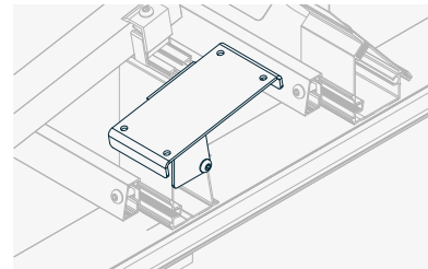
Halterung für Einstrahlungssensor zur Anbringung eines Einstrahlungssensors
